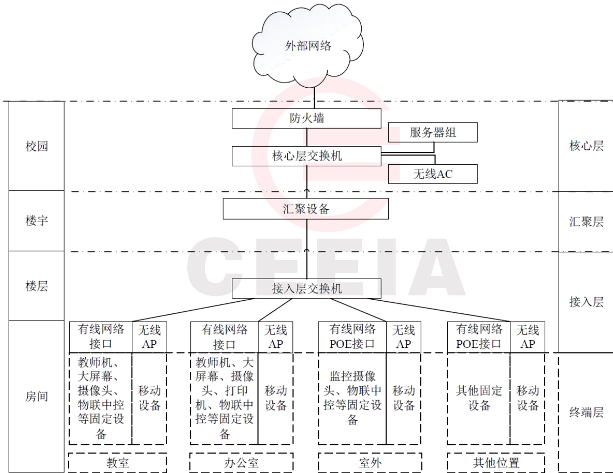
图 2 校园以太网架构
