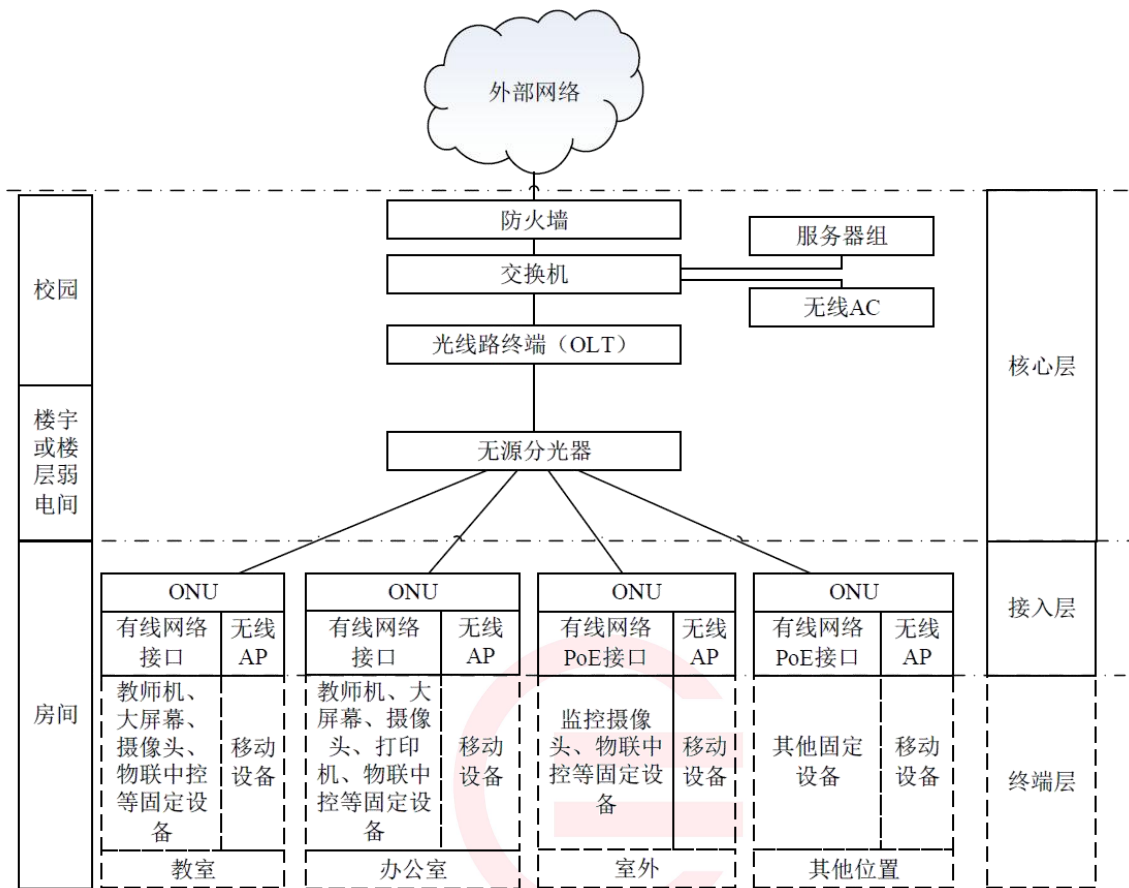
图3 校园无源光局域网架构
