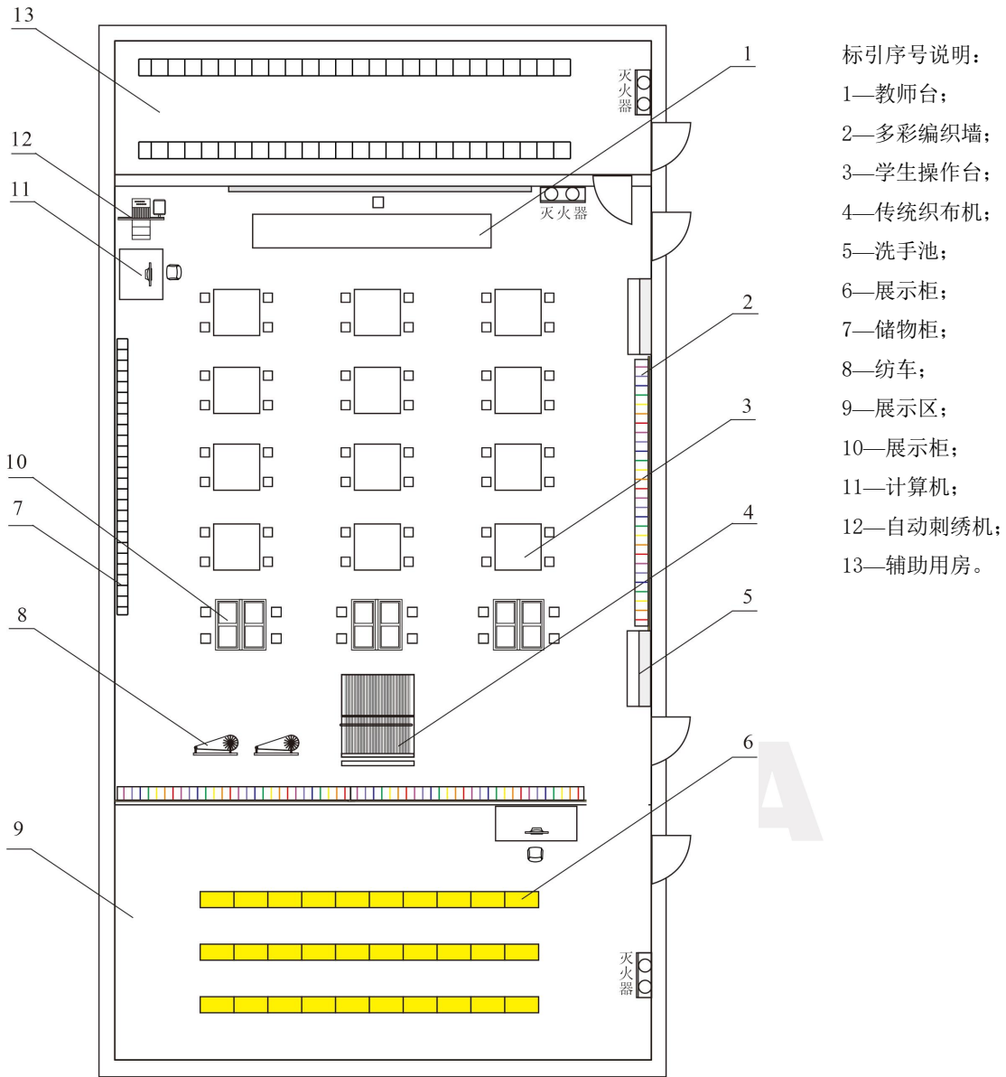
图 A.2 编织教室布置示意图（二）
